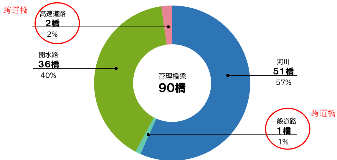
図 9 交差状況
